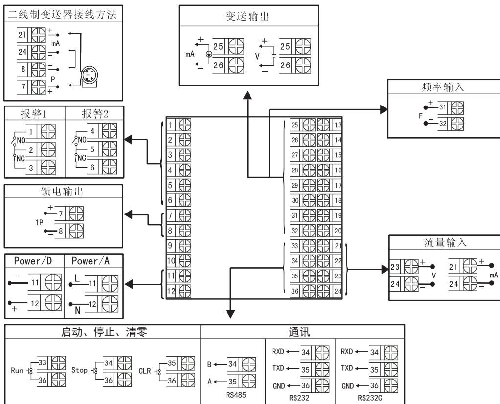
NHR-6602R接线图
