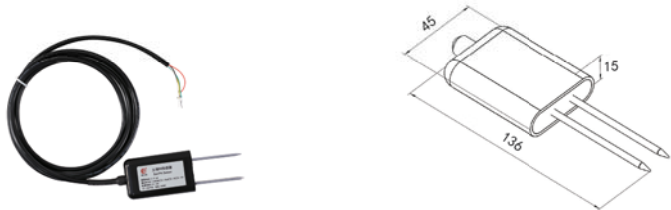
外形尺寸：45*15*136mm
