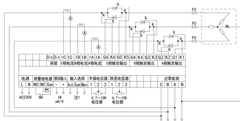
8、三相KP4（单向可控硅反并联，Y形接法星点接N）
