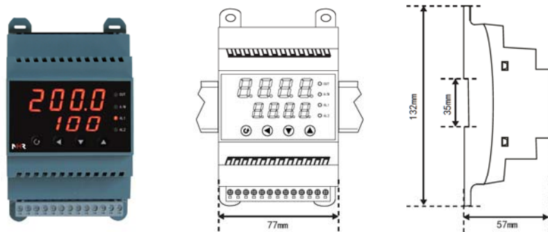
外形尺寸:宽*高*深:77×132×57mm
