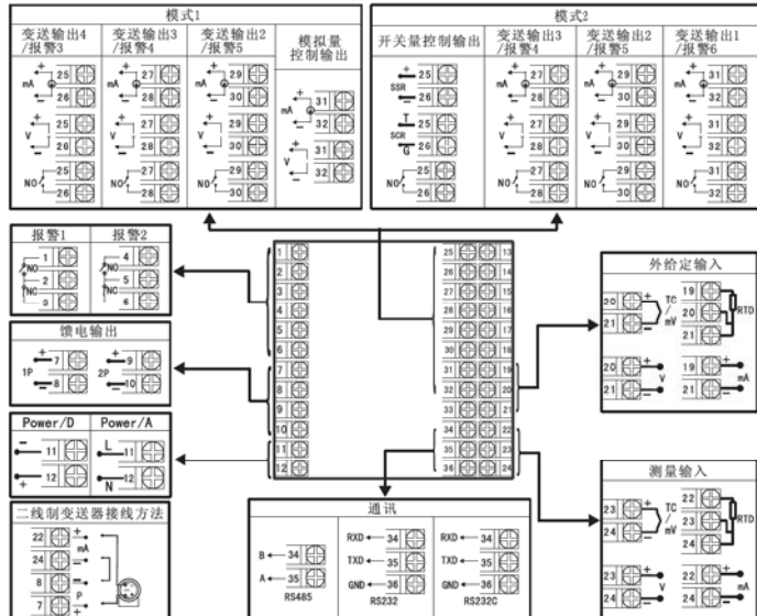
NHR-7320(R)系列仪表接线图
