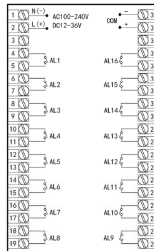
分别报警副机
