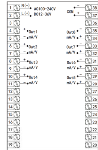
分别变送副机
