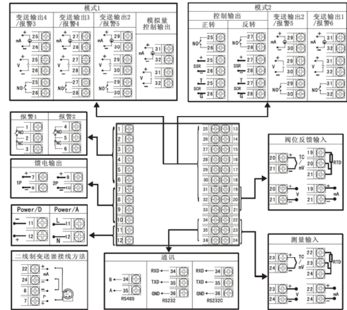
NHR-7330(R)系列仪表接线图
