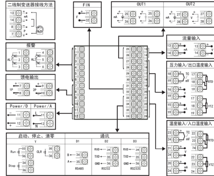
规格尺寸为A、B、C、D型接线图 注：横竖式仪表后盖接线端子方向不一样，见示意图1
