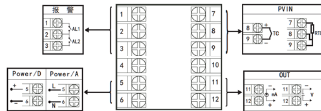
规格尺寸为H型接线图
