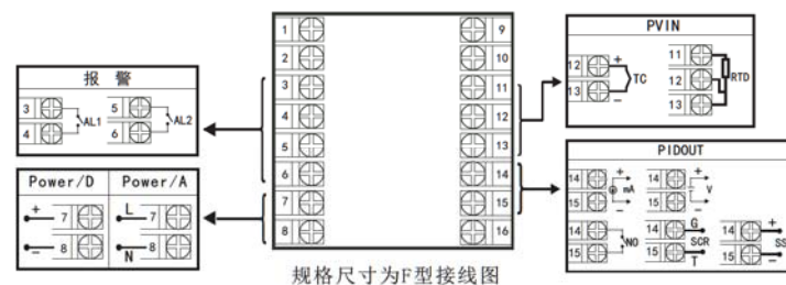
规格尺寸为F型接线图
