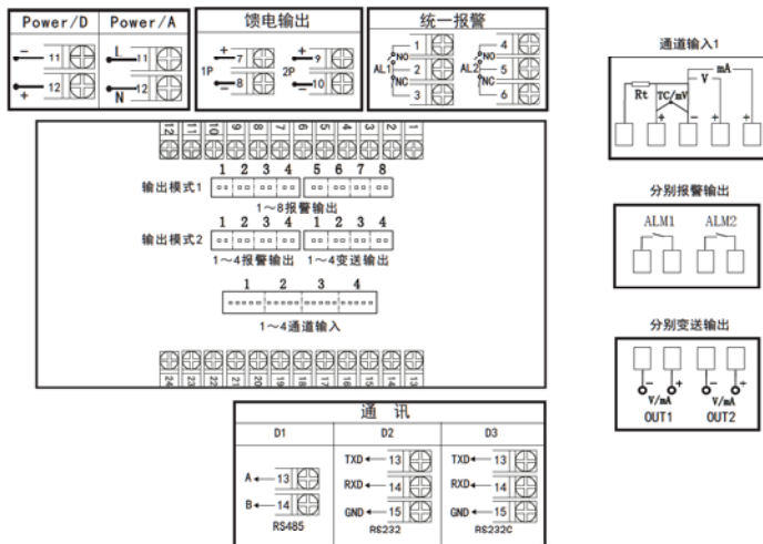
C型接线图
