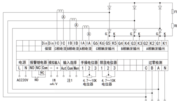
7、三相半控整流KZ3
