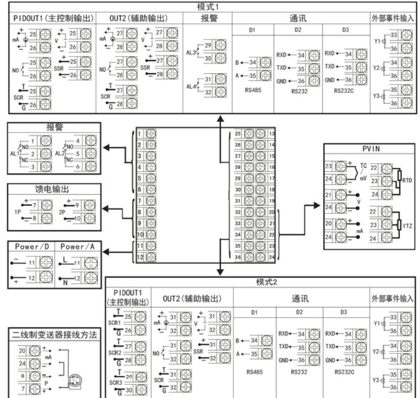
规格尺寸为A、B、C、D、E、K、L、M型接线图 注：横卧式仪表后盖接线端子方向不一样，见示意图1
