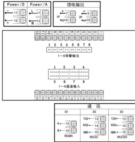
C型分别报警接线图
