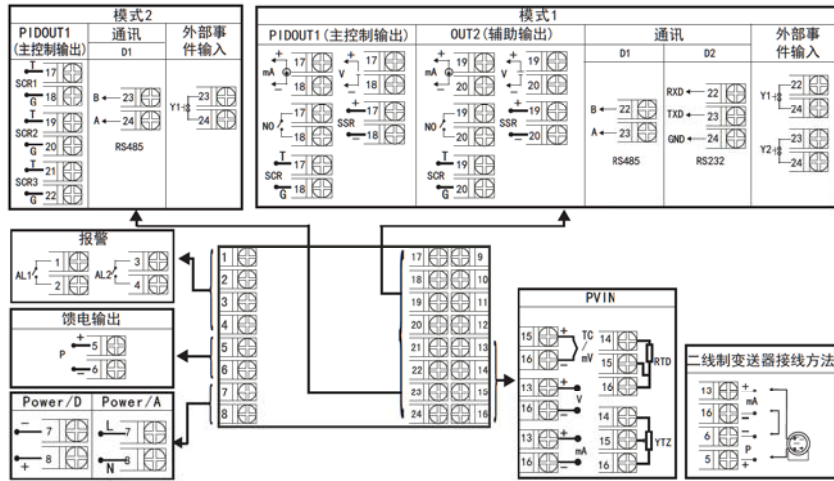
规格尺寸为F型接线图
