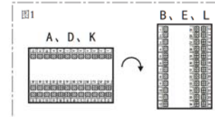
规格尺寸为A、B、C、D、E、K、L型接线图 注:横竖式仪表后盖接线端子方向不一样,见示意图1
