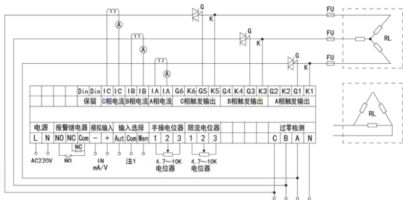
6、三相半控KY3（单向可控硅与整流管反并联，△形接法或Y形接法星点不接N）
