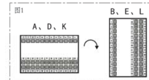
规格尺寸为A、B、C、D、E、K、L、M型接线图 注：横卧式仪表后盖接线端子方向不一样，见示意图1
