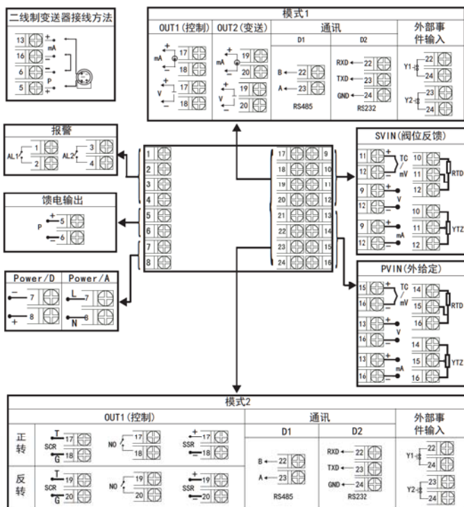
规格尺寸为F型接线图
