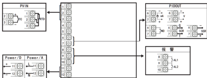
规格尺寸为C、D、E型接线图 注：横竖式仪表后盖接线端子方向不一样，见示意图1
