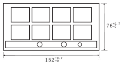
仪表开孔尺寸
