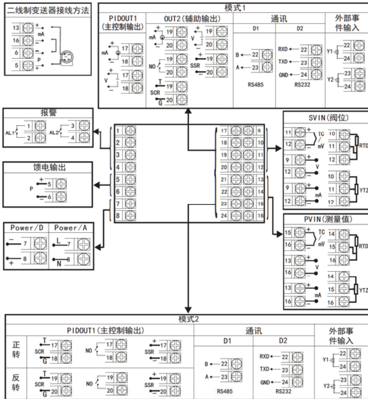
规格尺寸为F型接线图
