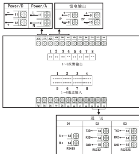
C型分别变送接线图
