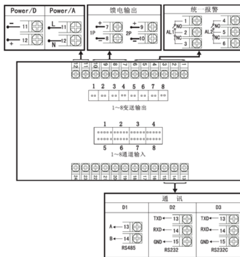
C型分别变送接线图
