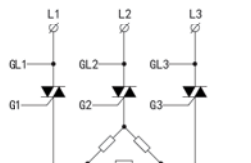
⑥、三角形三相三线制全控制结构 (单向可控硅反并联电路)
