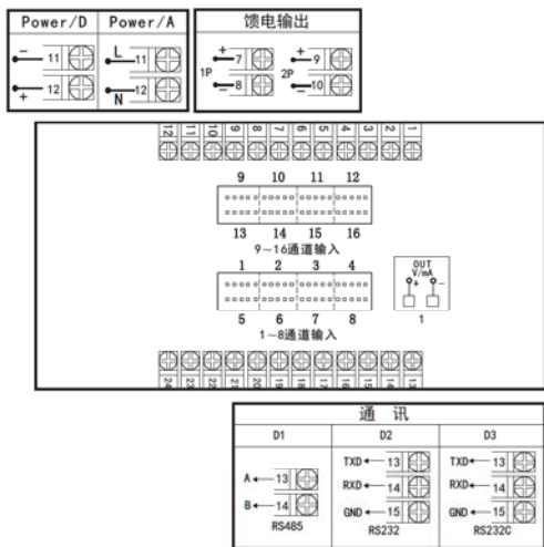
A、B型统一变送接线图
