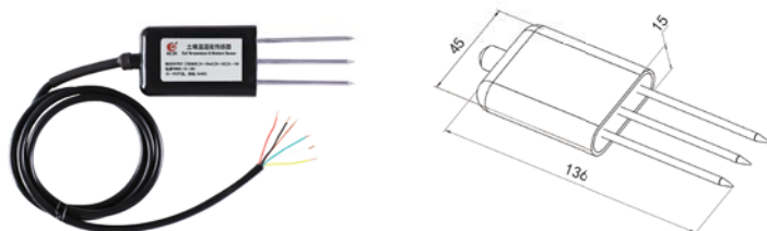
外形尺寸：45*15*136mm
