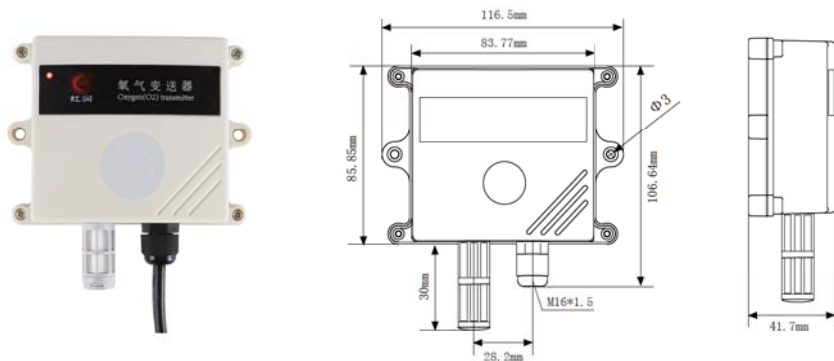
外形尺寸：宽*高*深：116.5×85.85×41.7mm
