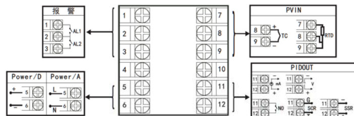
规格尺寸为H型接线图
