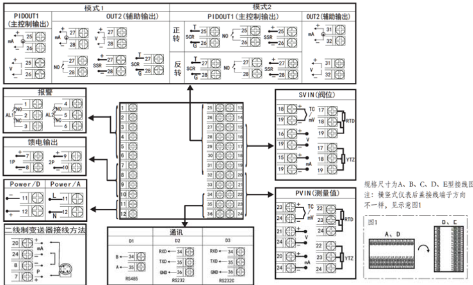
阀位反馈接线图
