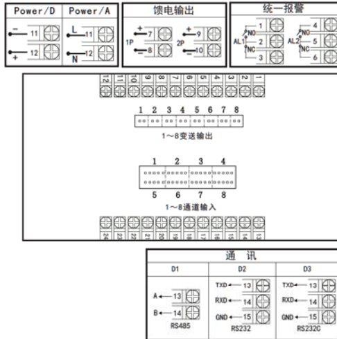
C型分别变送接线图
