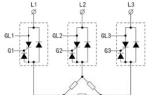
⑧、三角形三相三线制半控结构 (单向可控硅+二极管电路)
