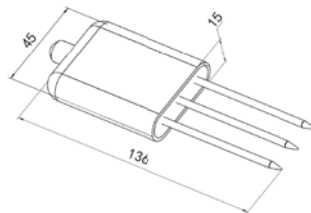
外形尺寸：45*15*136mm
