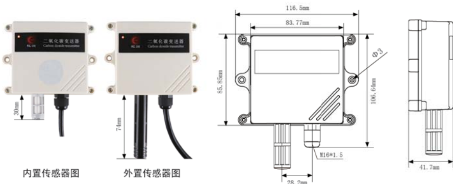
外形尺寸：宽*高*深：116.5×85.85×41.7mm
