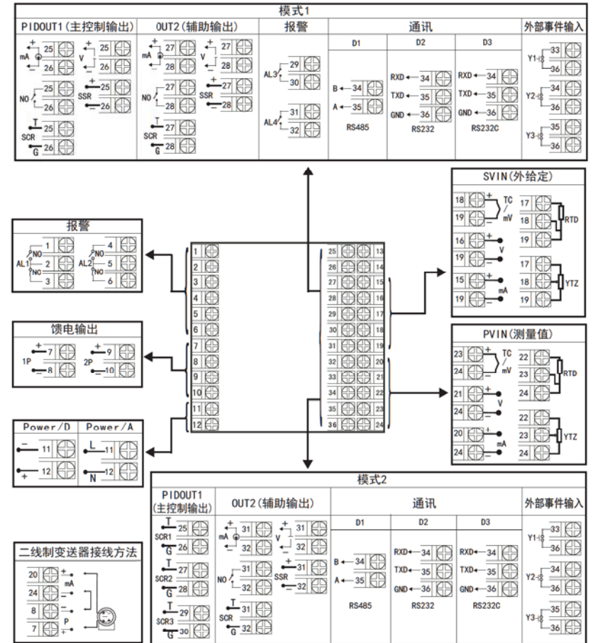
规格尺寸为A、B、C、D、E、K、L型接线图 注:横竖式仪表后盖接线端子方向不一样,见示意图1
