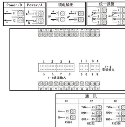
A、B型分别变送接线图
