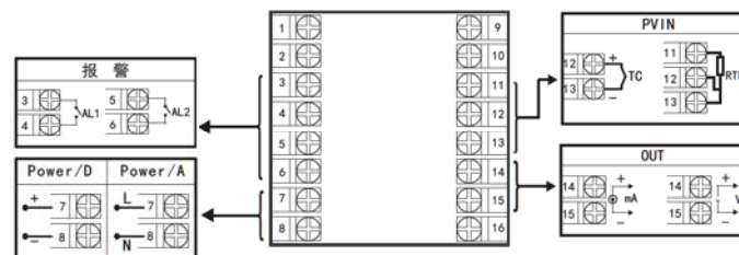
规格尺寸为F型接线图
