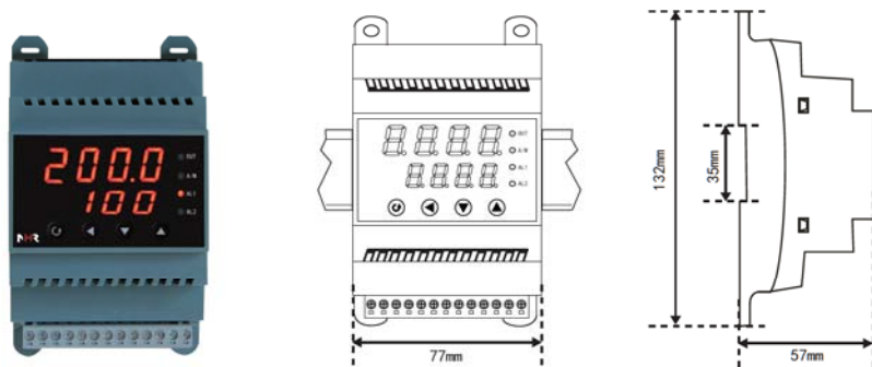
外形尺寸:宽*高*深:77×132×57mm
