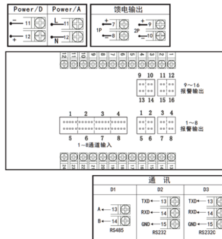
A、B型分别报警接线图
